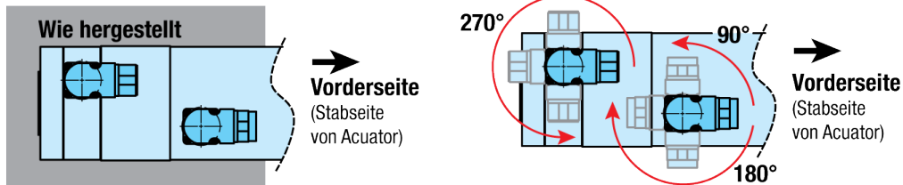
Abbildung 5.2: Steckerdrehung. Beachten Sie, dass die Tolomatic-Standardstecker von -90^\circ bis +180^\circ gedreht werden können, so dass die Kabel zur Vorderseite (Stangenende, wie hergestellt), zu einer Seite, zu beiden Seiten oder zur Rückseite des Aktuators angeschlossen werden können.
